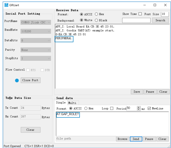
图 3-9 获取开发板B角色信息
