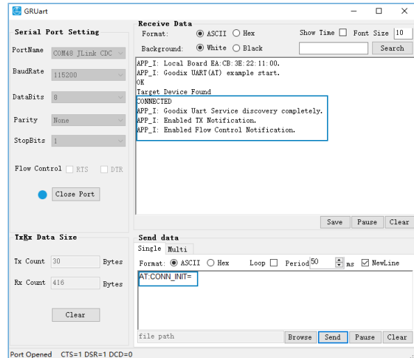
图 3-5 发现服务后发起连接
